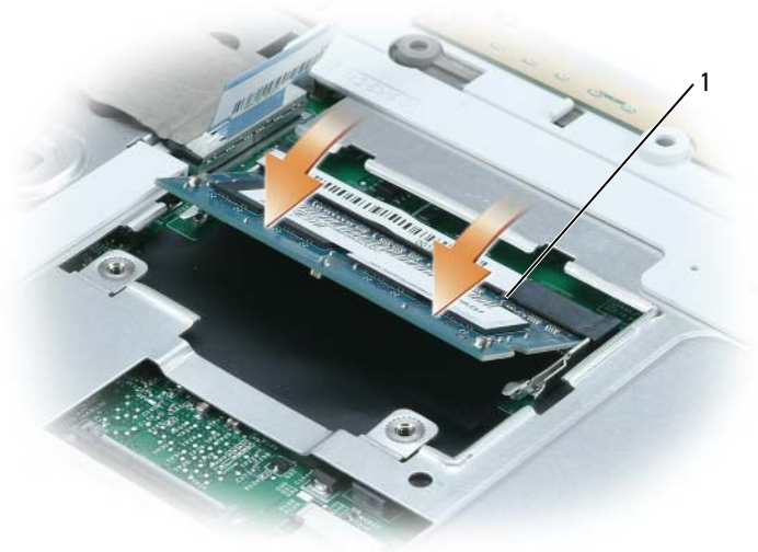
1 커넥터 슬롯에 있는 탭
