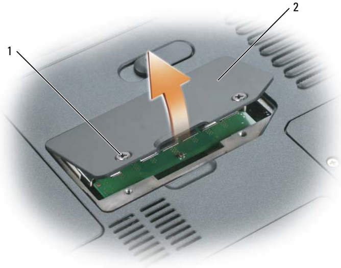
1 나사 (2 개)
