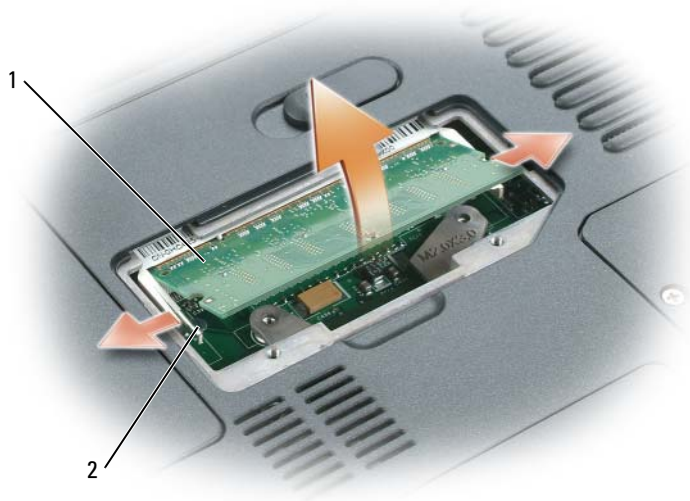
1 메모리 모듈
