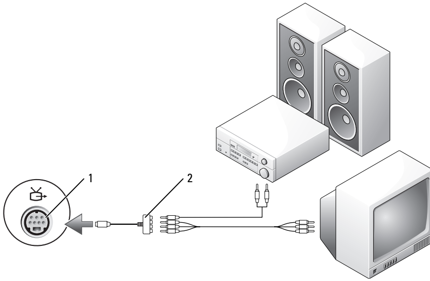
1 S-video TV-out 커넥터 2 구성요소 비디오 어댑터
