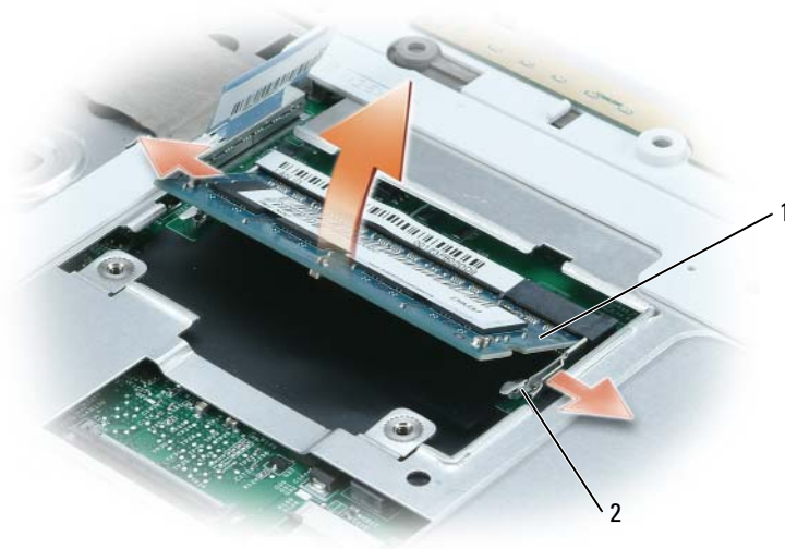
1 메모리 모듈
